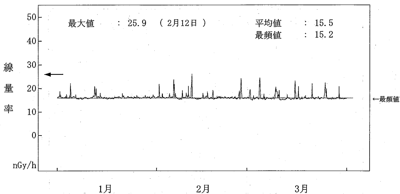
図－２－８ 空間ガンマ線線量率監視結果（塚浜局）
