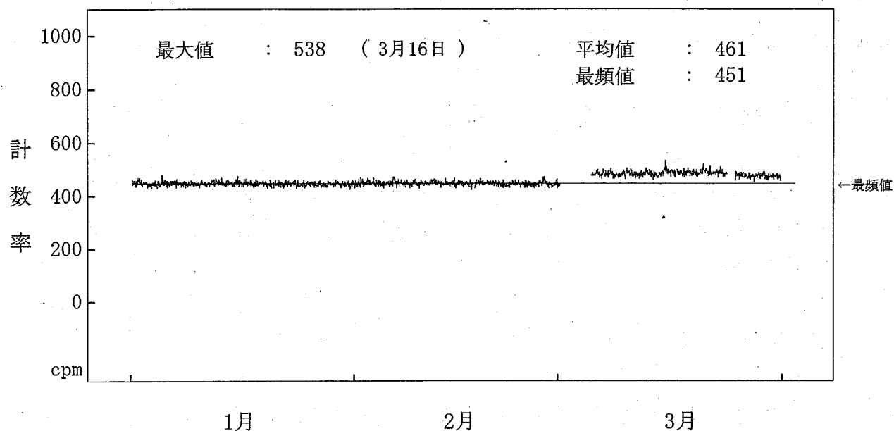
図－２－１４ 海水(放水)中の全ガンマ線計数率監視結果(3号機放水口モニター)
