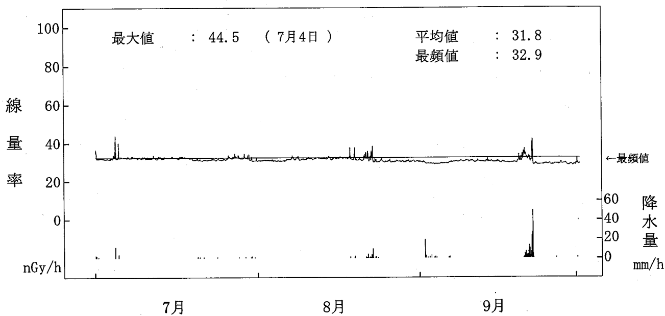
図－２－９ 空間ガンマ線線量率監視結果（寺間局）
