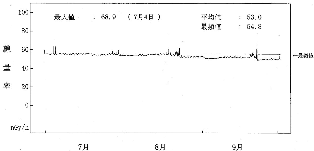
図－２－１１ 空間ガンマ線線量率監視結果（前網局）
