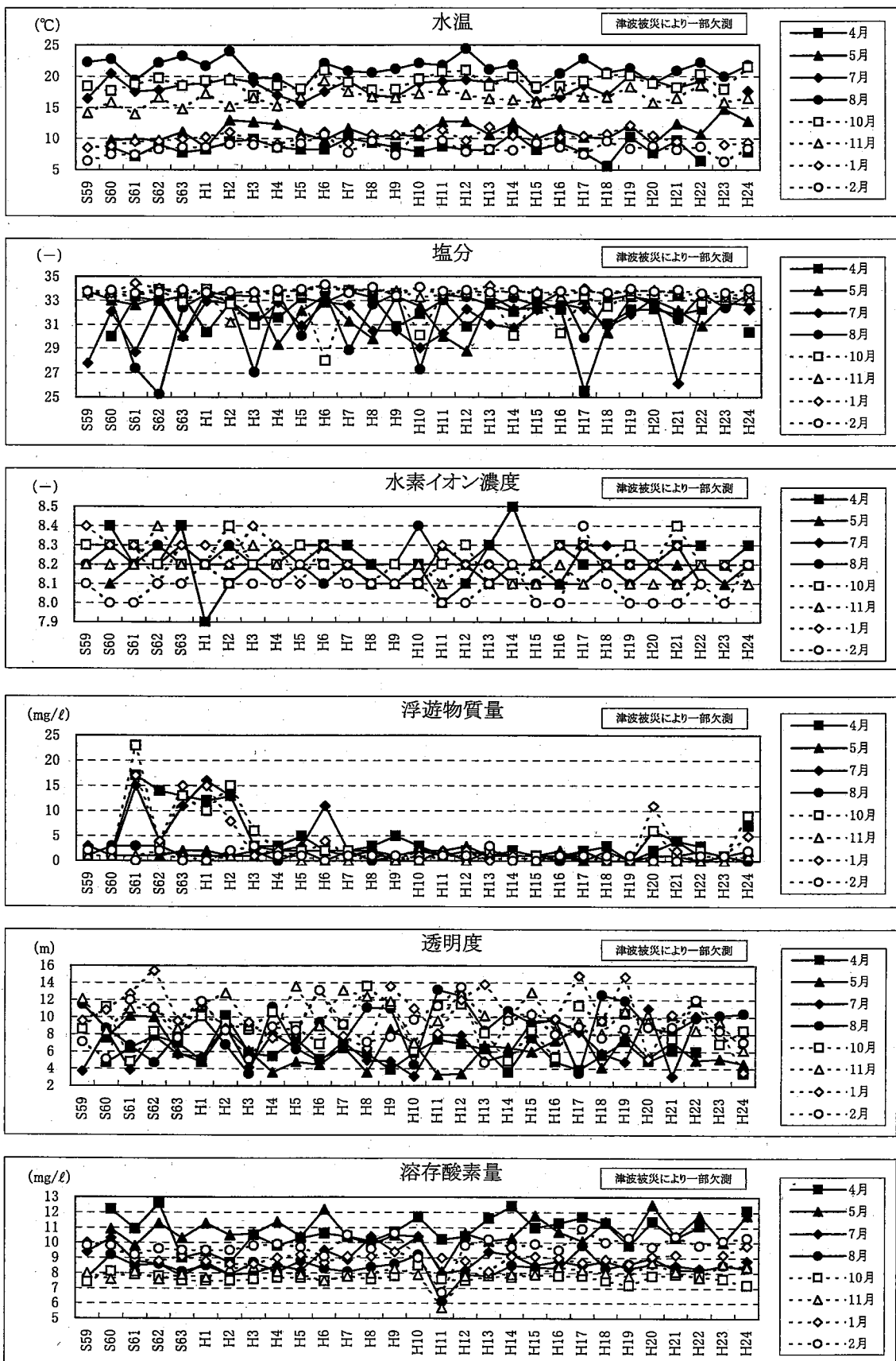
図Ⅲ-1-(2) 水質(海面下0.5m層)の月別経年変化
