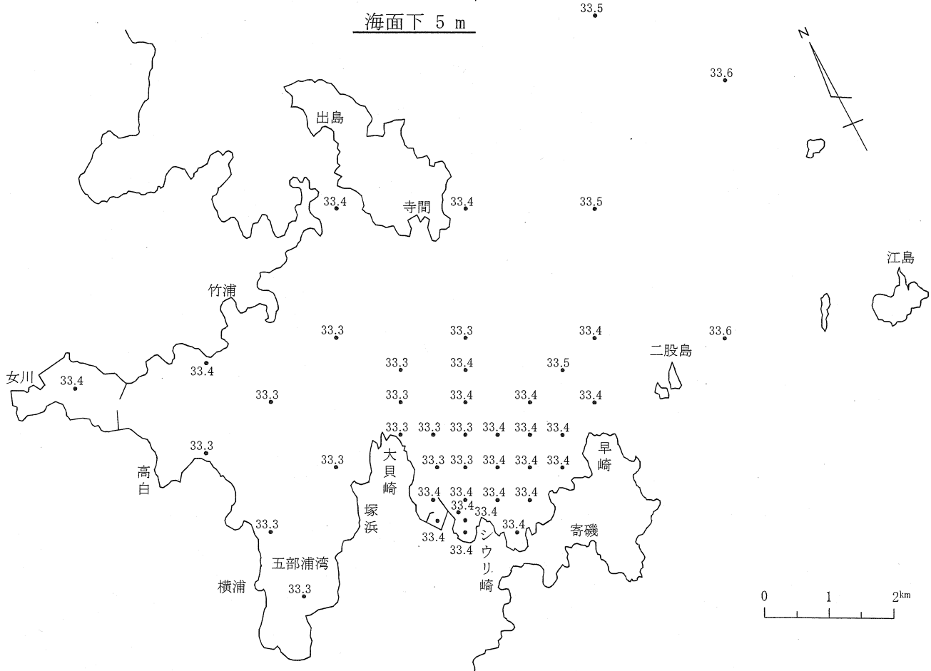
図-13-(1) 塩分水平分布
