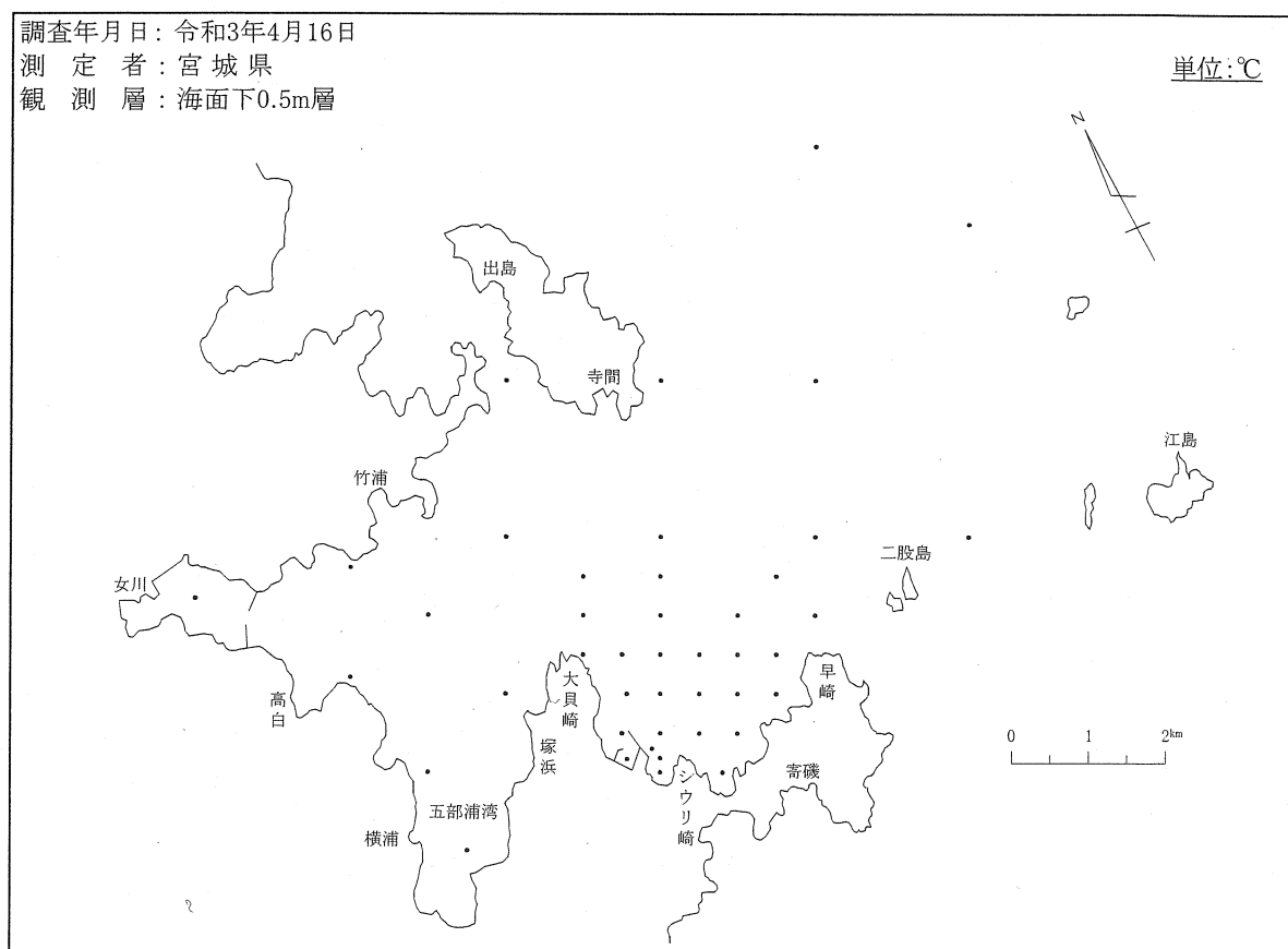
図－2－(2) 等温線
