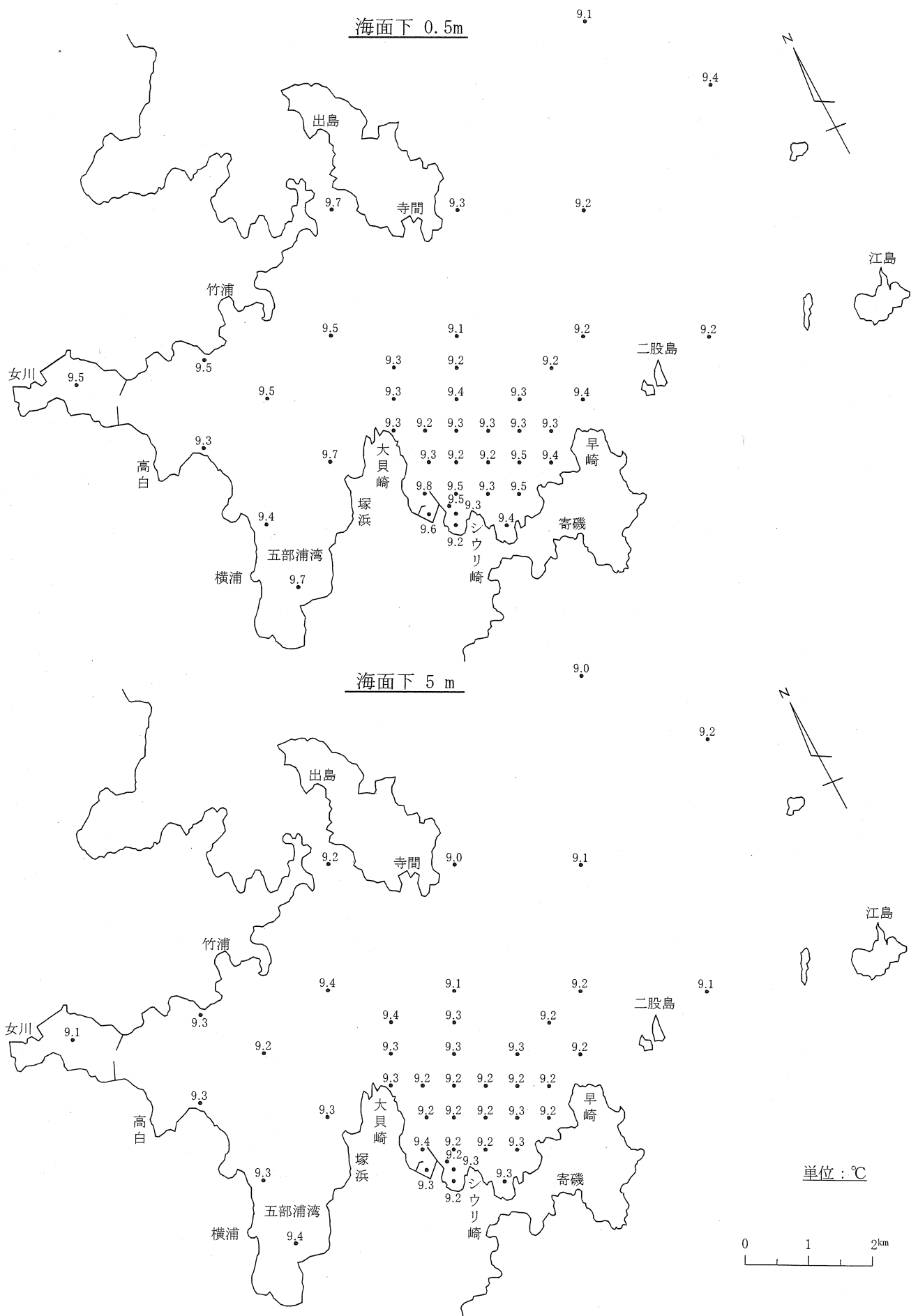
図-11-(1) 水温水平分布
