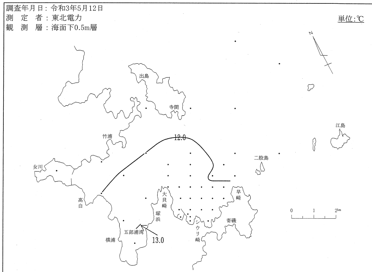
図－4－(2) 等温線
