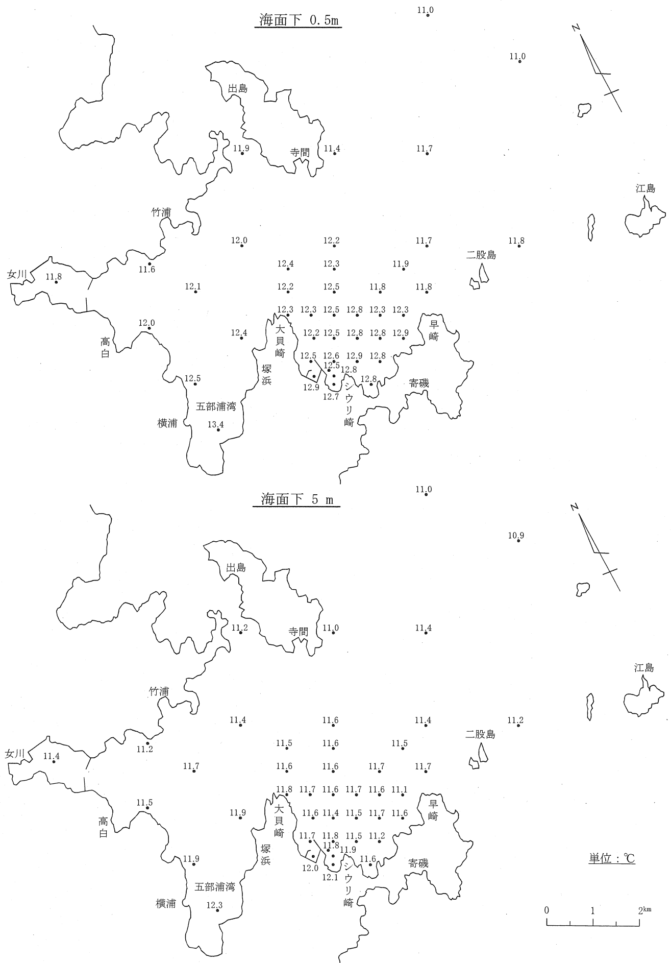
図-12-(1) 水温水平分布
