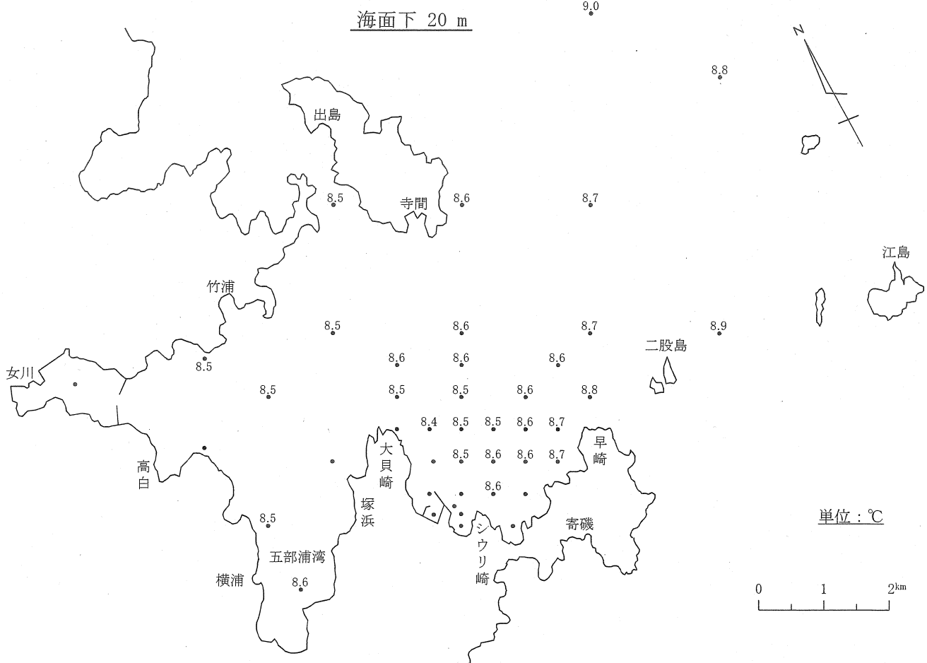
図-11-(2) 水温水平分布
