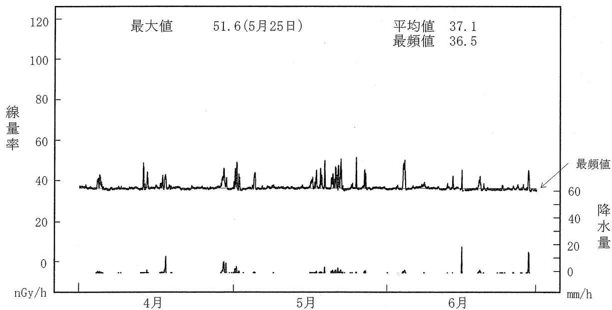
図－２－４ 空間ガンマ線量率監視結果（寄磯局）
