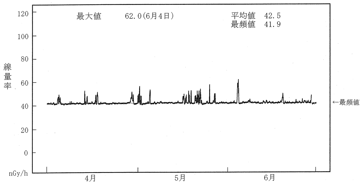
図－２－２ 空間ガンマ線量率監視結果（飯子浜局）
