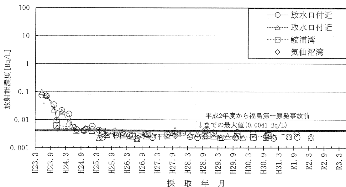
図-2-25 海水のCs-137濃度の推移
