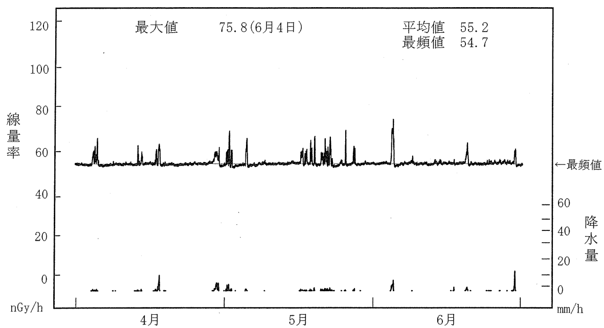
図－２－７ 空間ガンマ線量率監視結果（荻浜局）
