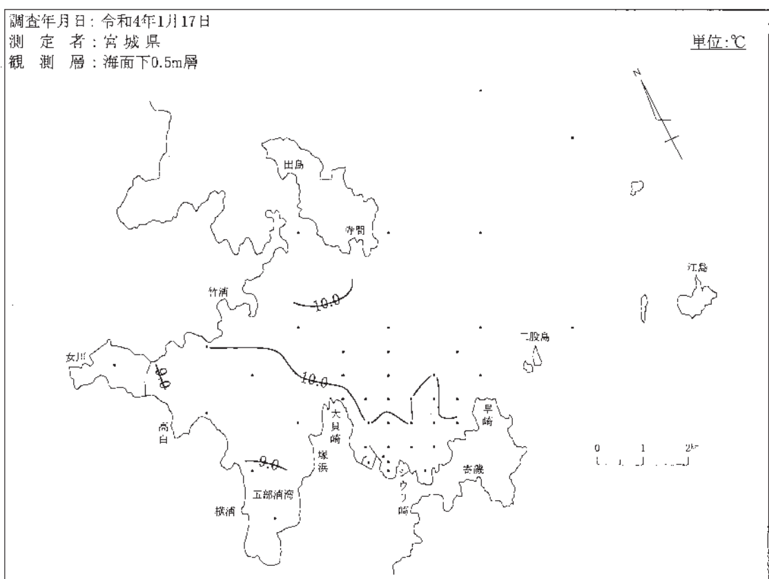
図-2-(2) 等温線
