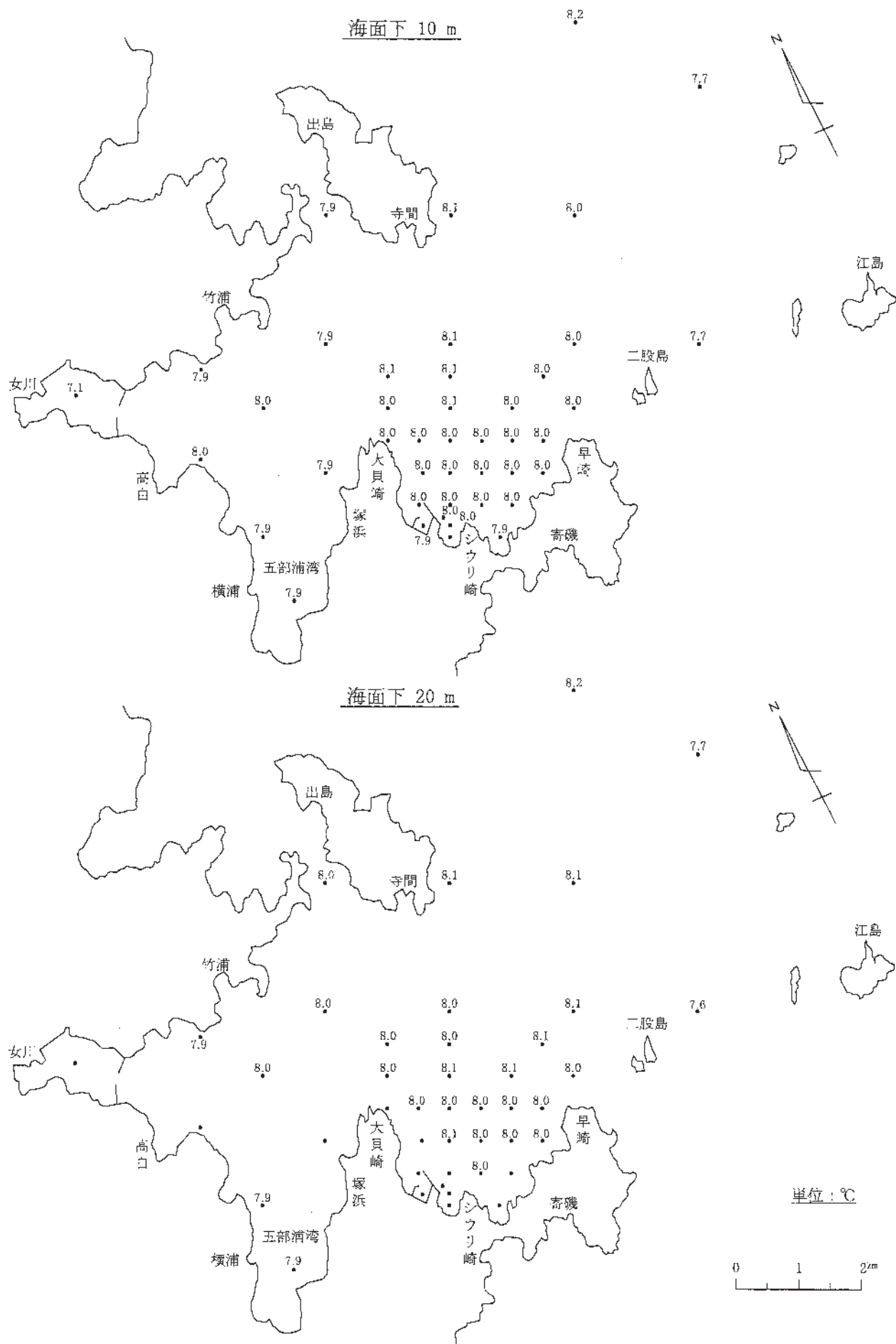
図-12-(2) 水温水平分布
