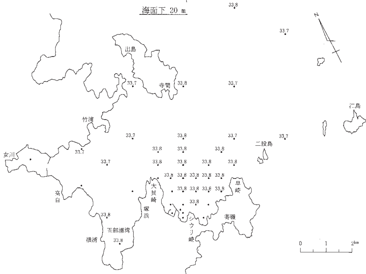
図－14－(2) 塩分水平分布
