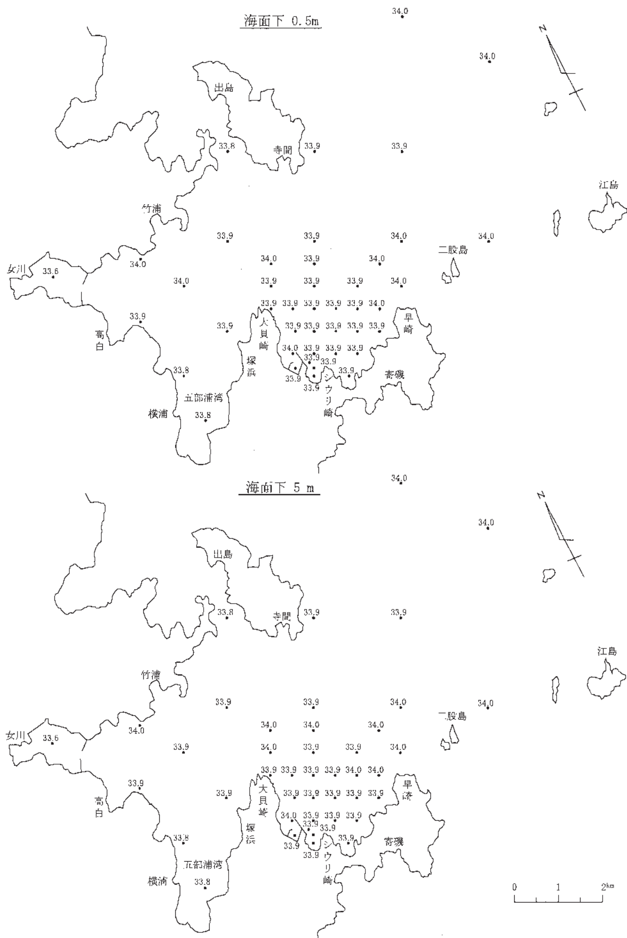
図-13-(1) 塩分水平分布
