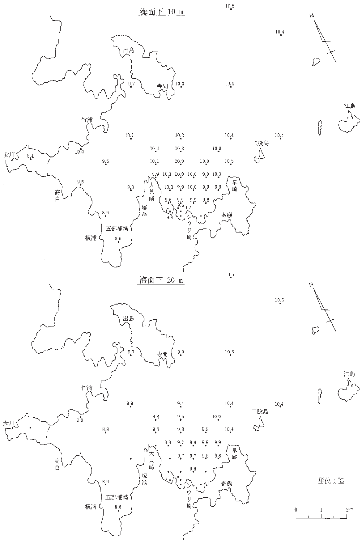
図一11-(2) 水温水平分布
