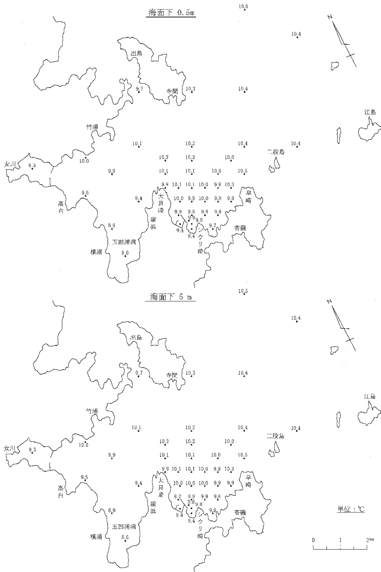
図－11－(1) 水温水平分布
