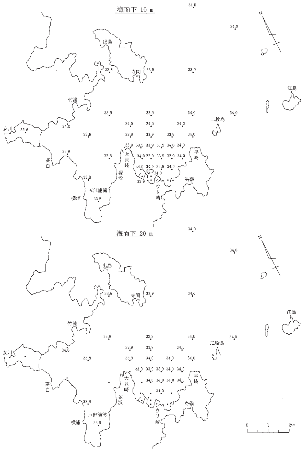
図-13-(2) 塩分水平分布
