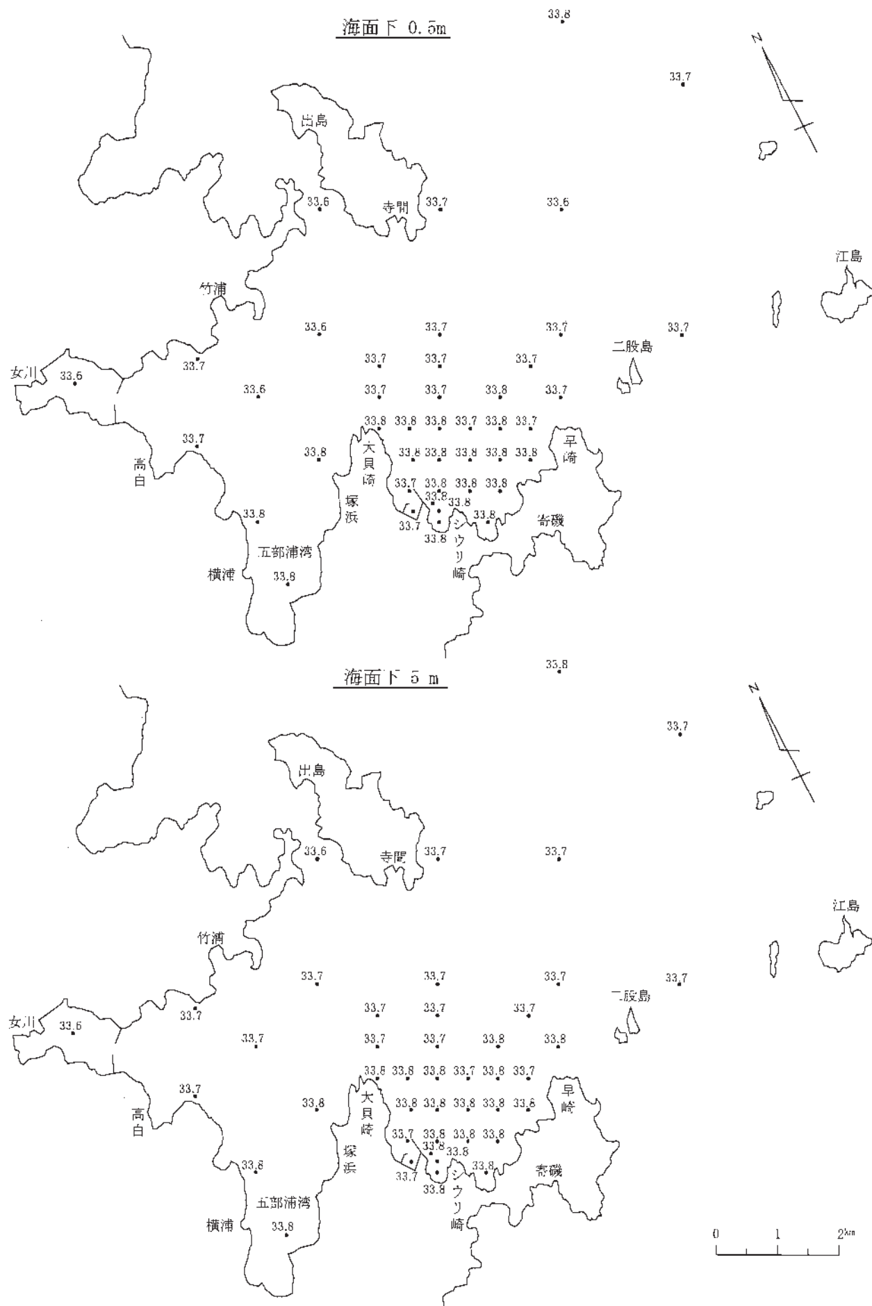
図－14－(1) 塩分水平分布
