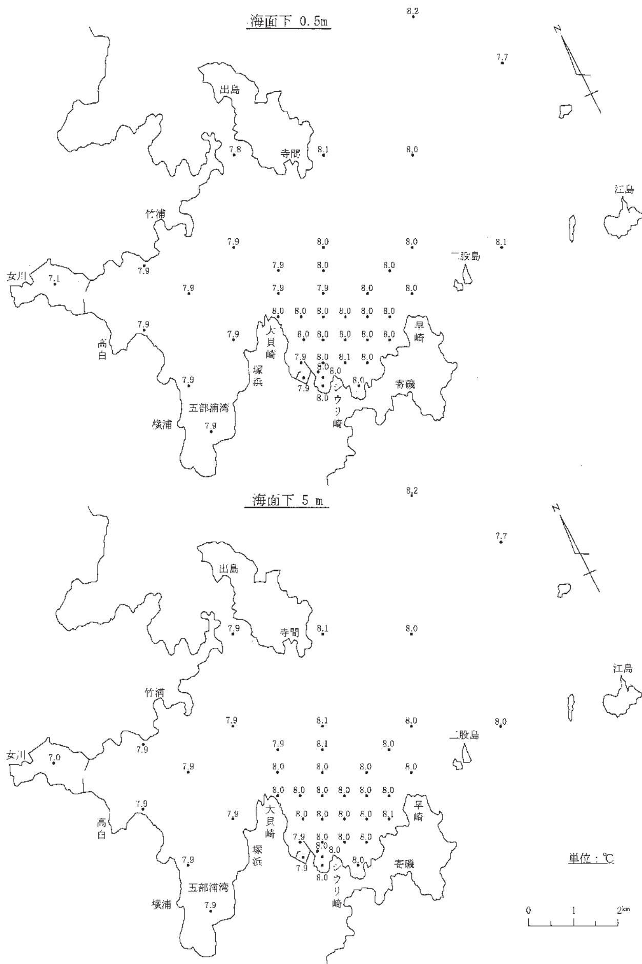
図一12-(1) 水温水平分布
