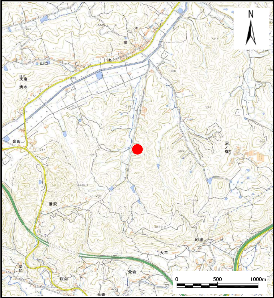
位置図(S=1:25,000)
